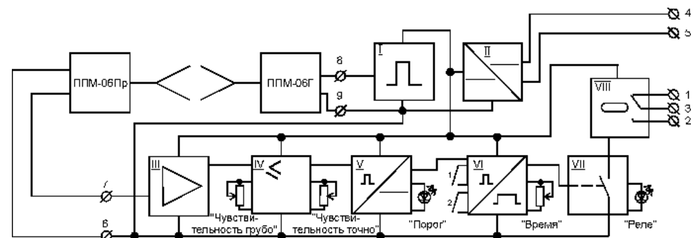
Рис. 2. Структурная схема датчика РСУ-6.
